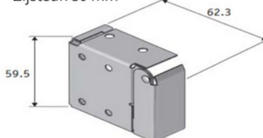
Zijsteun 50 mm
