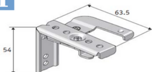
Beugel 35 - 50 - 70 mm
