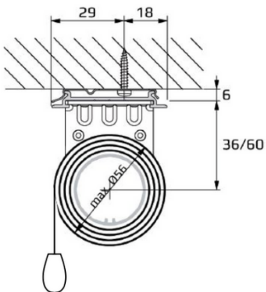
Plafondmontage
