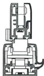
Geïntegreerde waterafvoer
