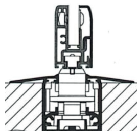
Verzonken
